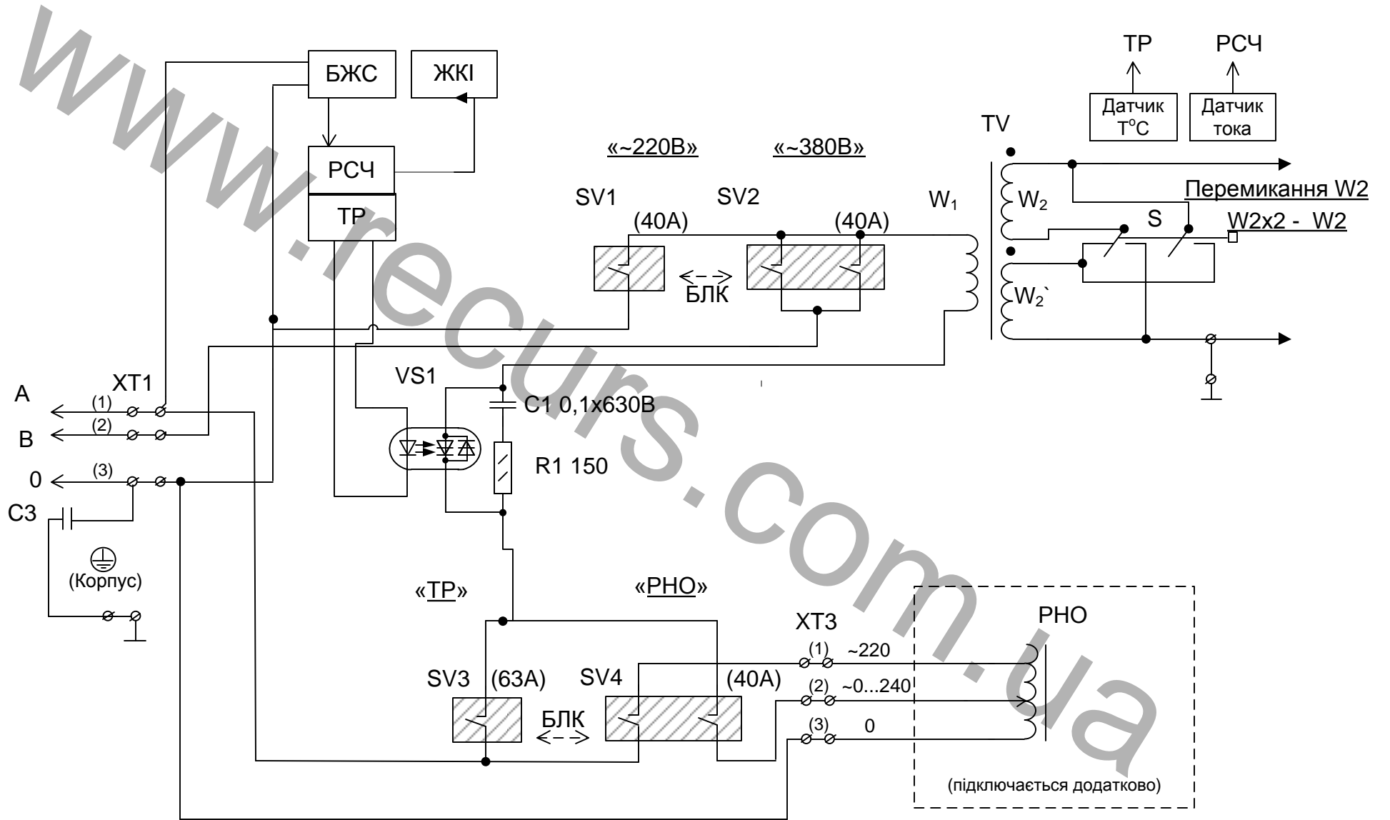
Рис.1 Функціональна схема УПА-10Р
